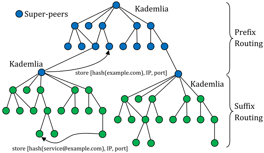
Fig. 6. Hierarchical Kademlia Overlay Network
